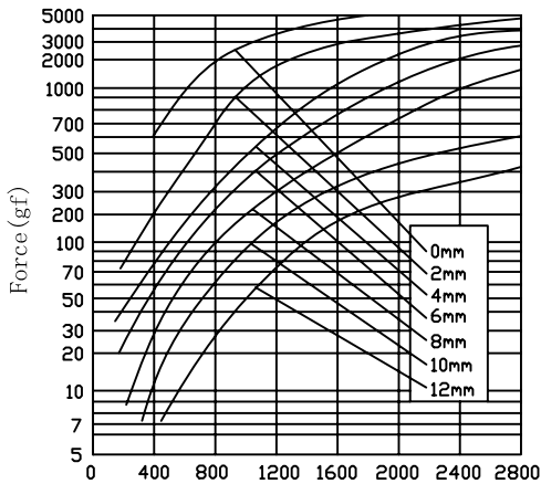
AMPERE-TURNS Vs FORCE 安匝/吸引力
